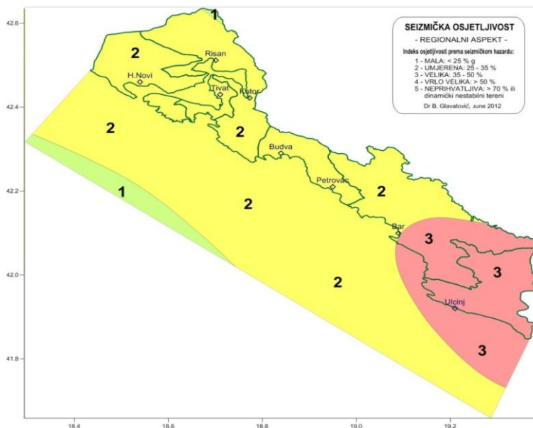
Slika 2.4. Karta matrice indeksa opšte (regionalne) seizmičke kategorizacije prostora Studija seizmičke mikrorejionizacije za primorske opštine, prof.dr. Glavatović B., Vučinić Lj., dipl.matemat., CAMP CG, februar 2013. g.
