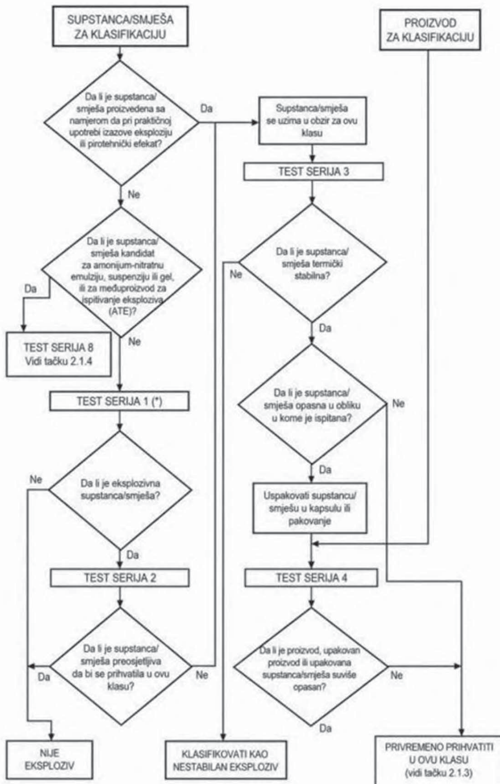
Slika 2.1.3. Postupak klasifikacije u jednu od podklase klase eksploziva (Klasa 1 za transport opasnog tereta)
