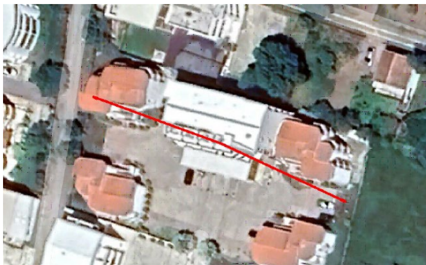
Pozicija antenskih nosača sa prikazanim azimutima Mtel antena, graničnom zonom i okolnim objektima
