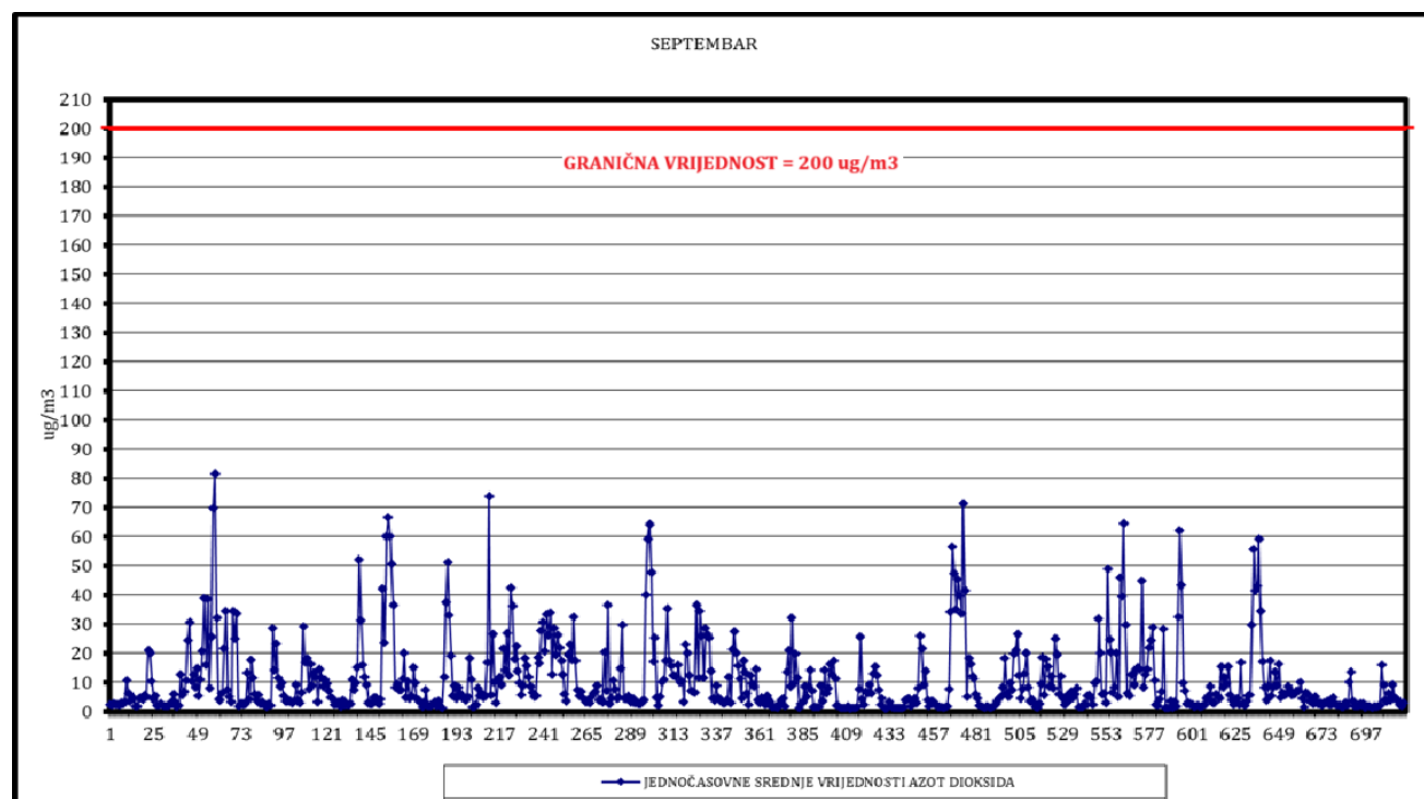
Slika 6. Jednočasovne srednje vrijednosti azot dioksida
