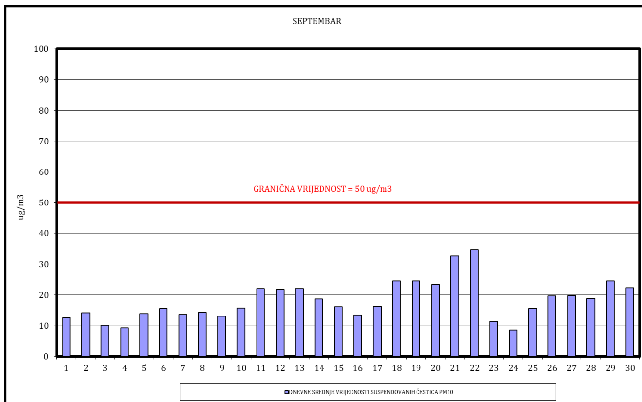
Slika 14. Dnevne srednje vrijednosti suspendovanih čestica PM 10
