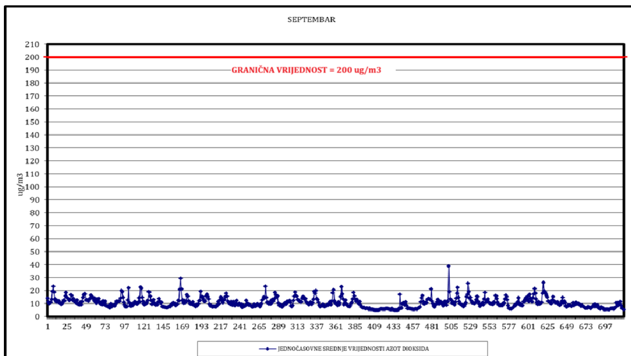
Slika 12. Jednočasovne srednje vrijednosti azot dioksida
