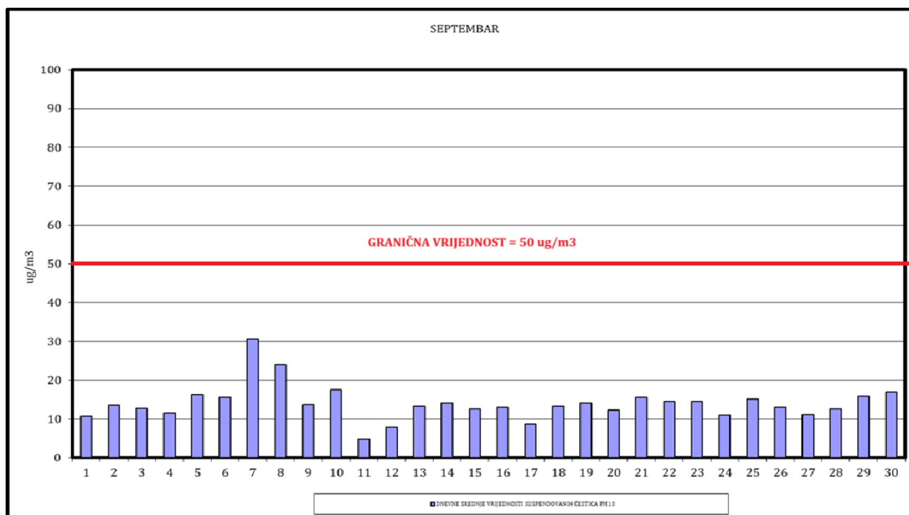
Slika 8. Dnevne vrijednosti suspendovanih čestica PM 10
