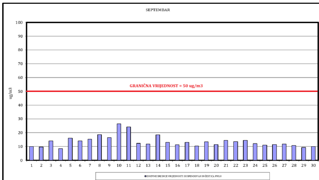
Slika 16. Dnevne srednje vrijednosti suspendovanih čestica
