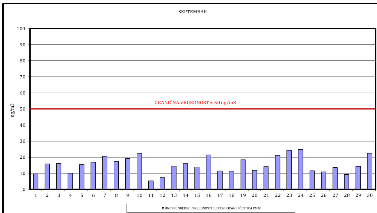
Slika 1. Dnevne srednje vrijednosti suspendovanih čestica PM 10
