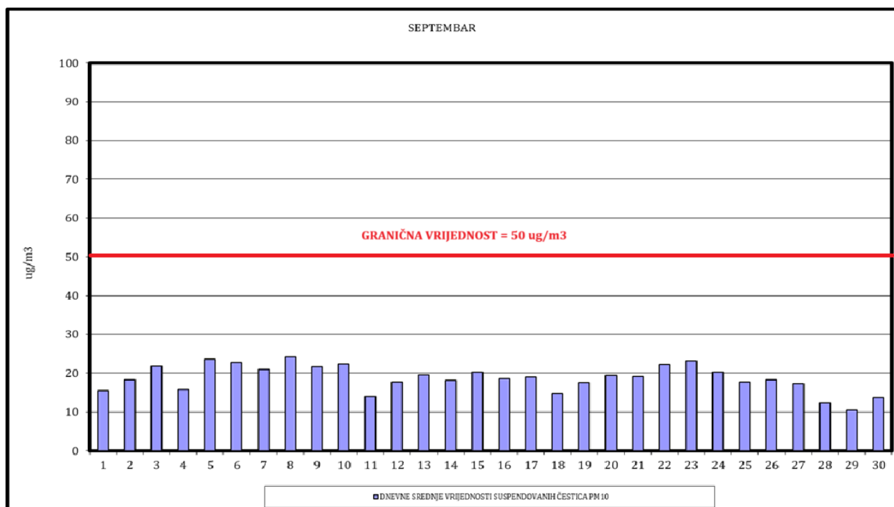
Slika 9. Dnevne srednje vrijednosti suspendovanih čestica PM 10
