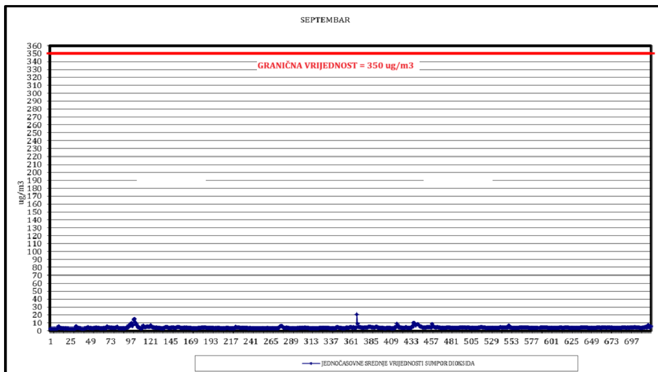
Slika 15. Jednočasovne srednje vrijednosti sumpor dioksida
