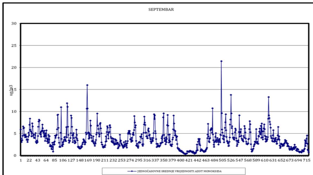
Slika 11. Jednočasovne srednje vrijednosti azot monoksida
