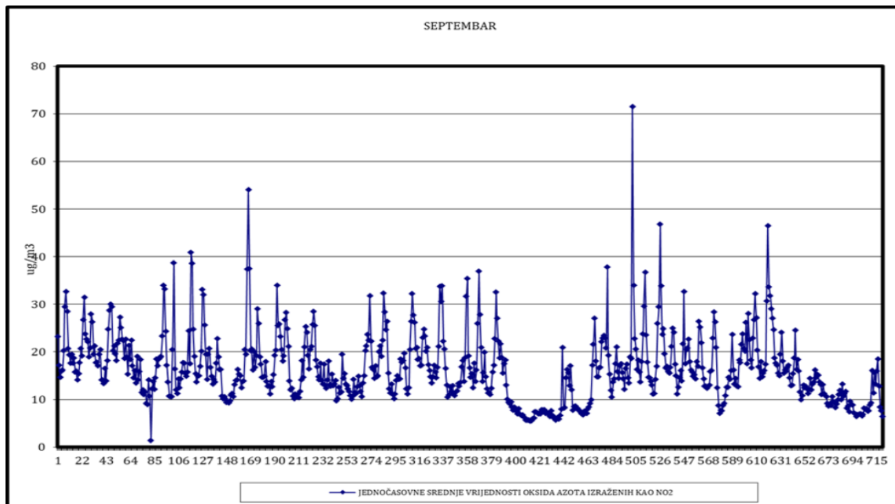
Slika 13. Jednočasovne srednje vrijednosti ukupnih oksida azota
