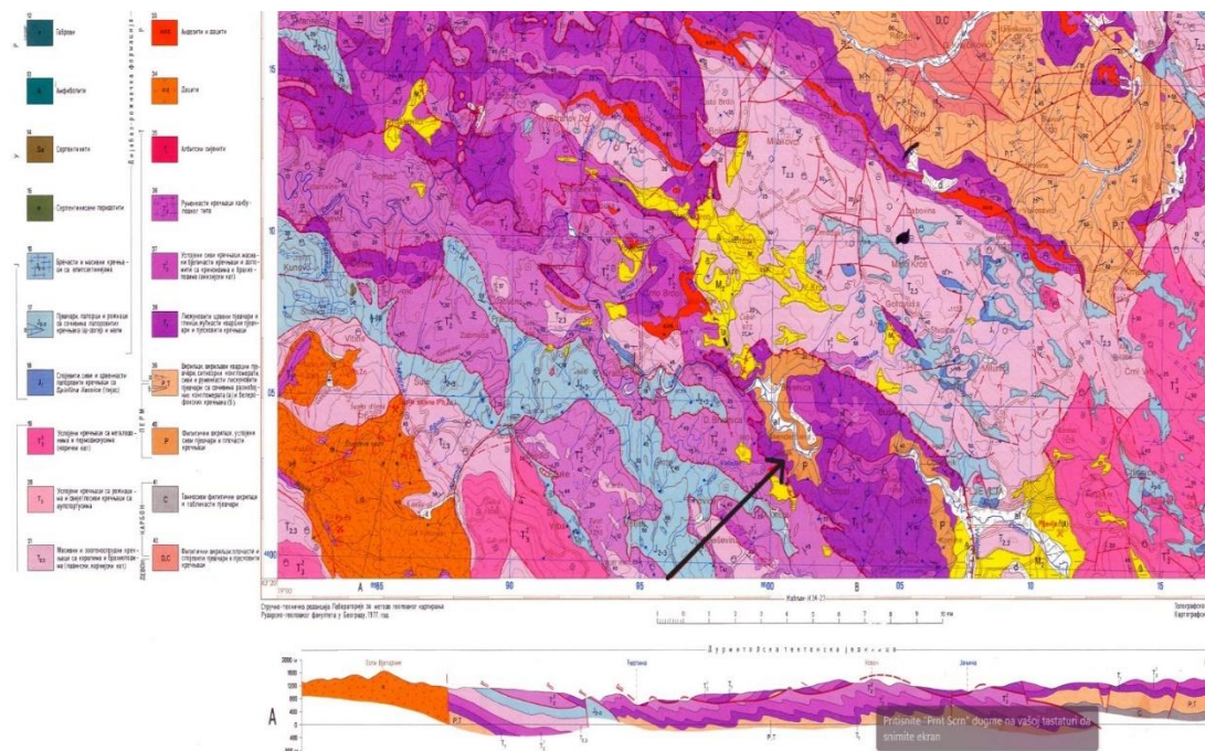
Slika 2.2. Geološka karta sa prikazom tačne lokacije predmetnog područja i legendom (Geološka karta SFRJ 1:1000000)
