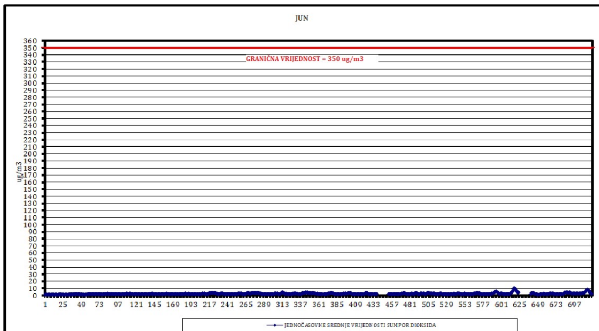
Slika 20. Jednočasovne srednje vrijednosti sumpor dioksida
