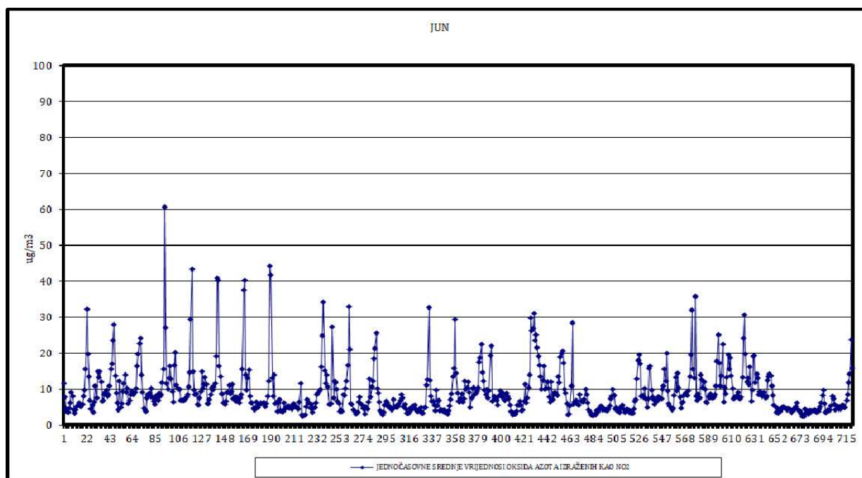
Slika 28. Jednočasovne srednje vrijednosti ukupnih oksida azota
