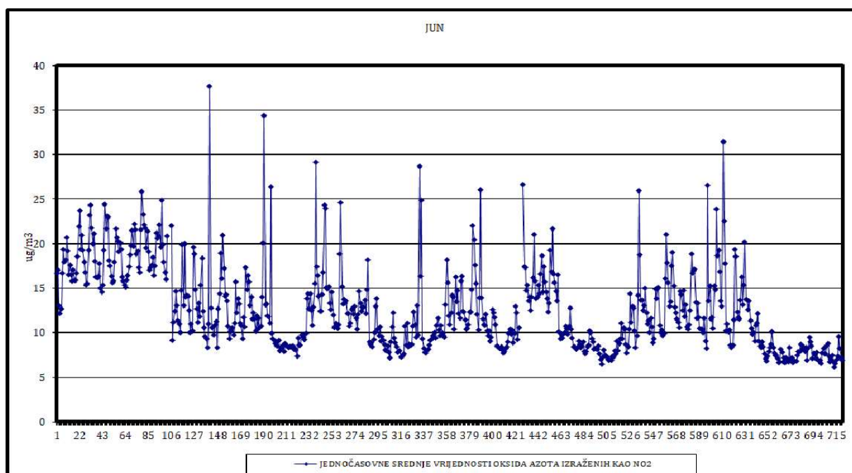
Slika 23. Jednočasovne srednje vrijednosti ukupnih oksida azota
