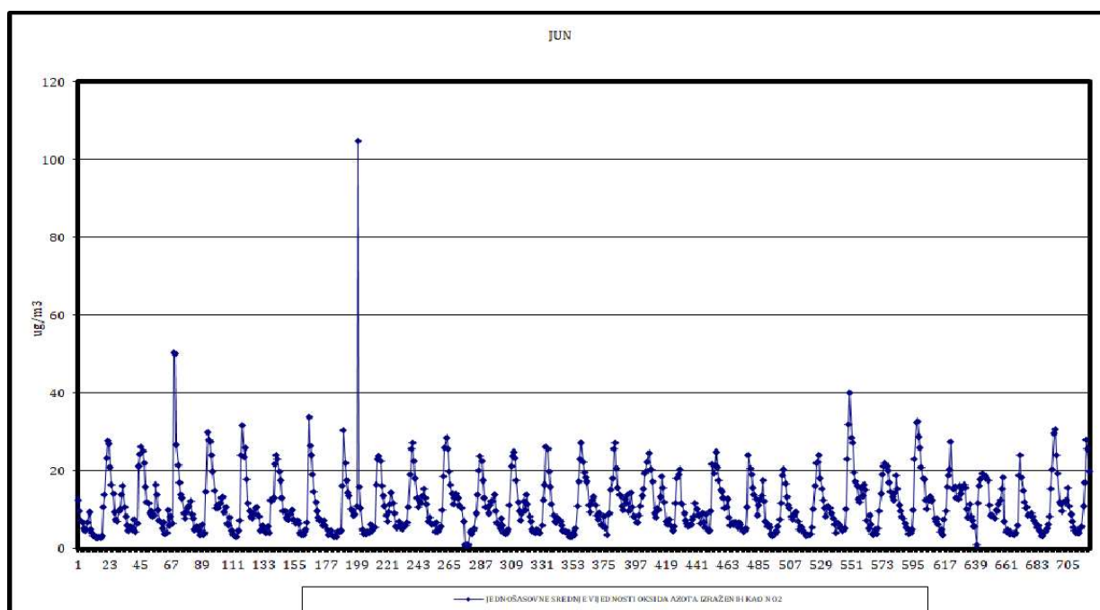
Slika 14. Jednočasovne srednje vrijednosti ukupnih oksida azota
