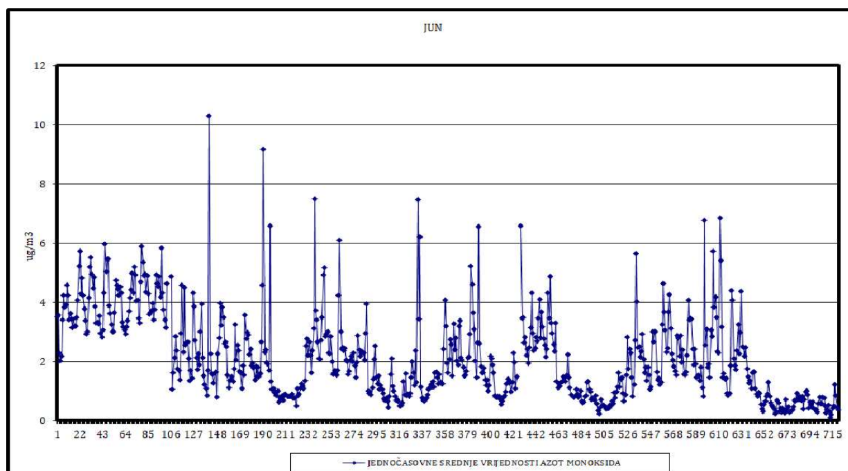
Slika 21. Jednočasovne srednje vrijednosti azot monoksida
