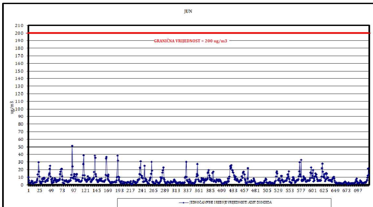
Slika 27. Jednočasovne srednje vrijednosti azot dioksida
