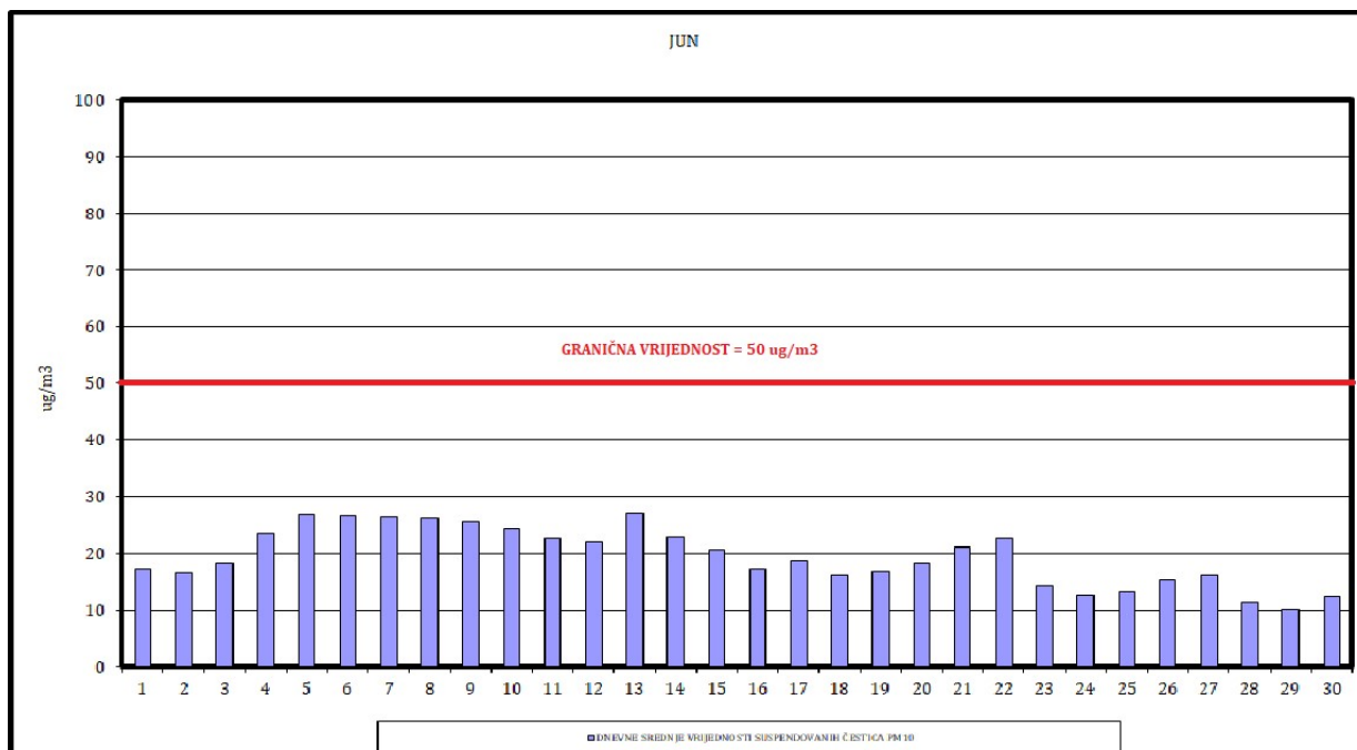
Slika 11. Dnevne vrijednosti suspendovanih čestica PM 10
