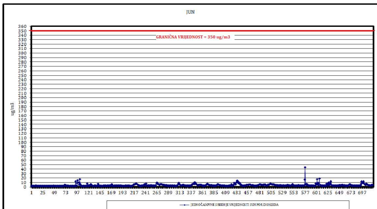
Slika 25. Jednočasovne srednje vrijednosti sumpor dioksida
