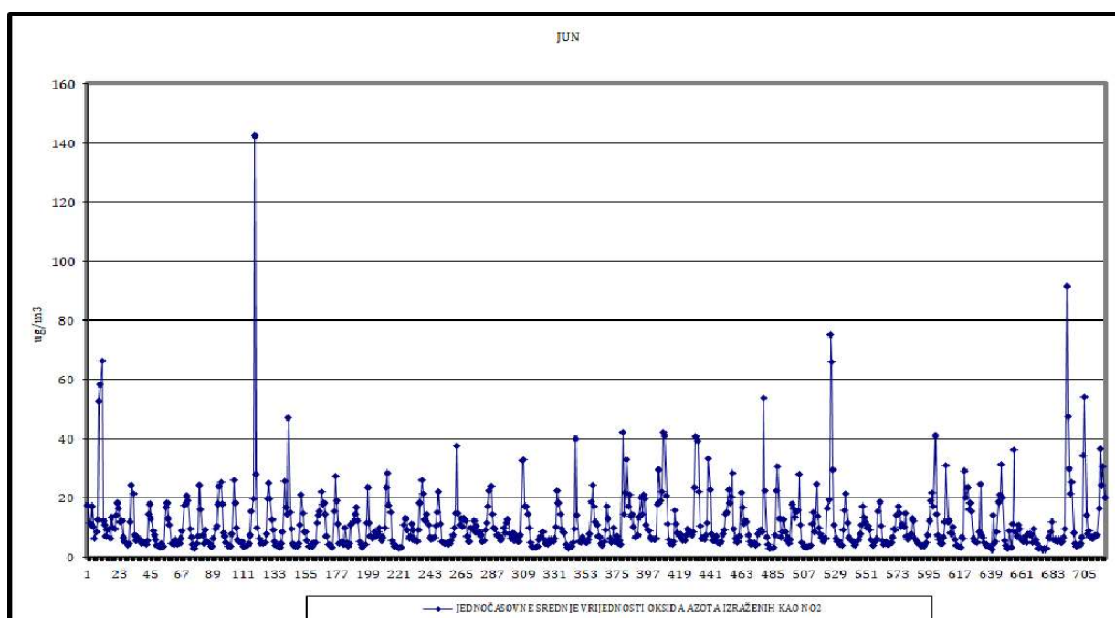
Slika 32. Jednočasovne srednje vrijednosti ukupnih oksida azota
