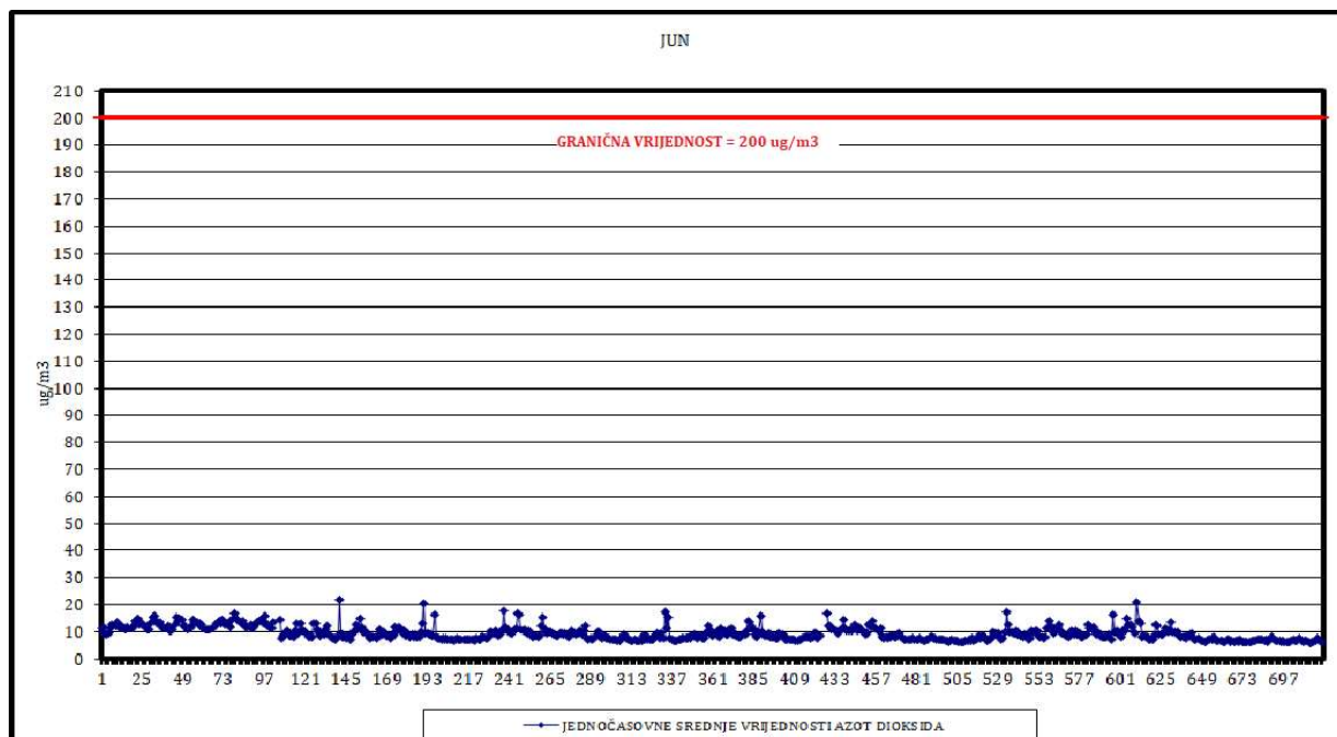
Slika 22. Jednočasovne srednje vrijednosti azot dioksida
