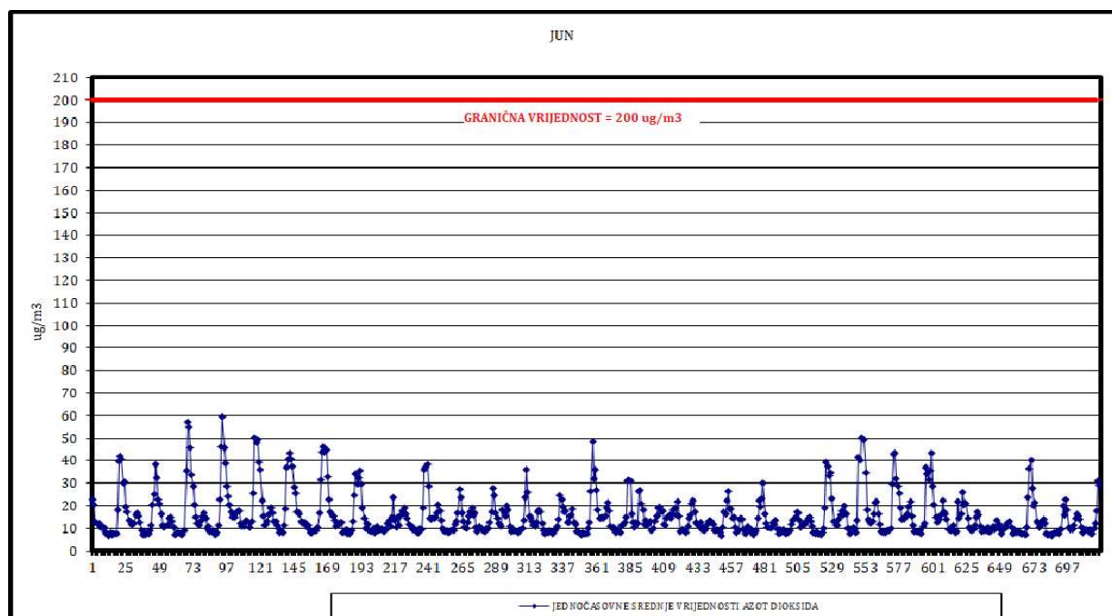
Slika 5. Jednočasovne srednje vrijednosti azot dioksida
