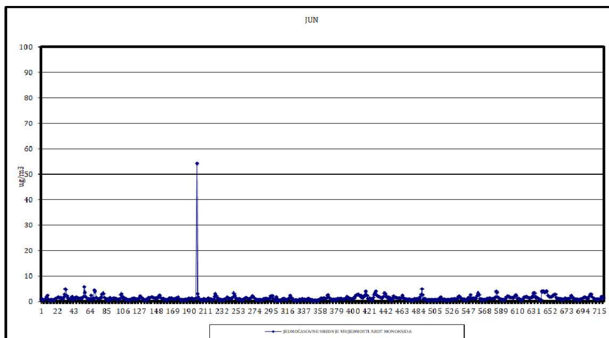
Slika 12. Jednočasovne srednje vrijednosti azot monoksida
